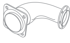
Артикул 120-14-062 Наименование Труба выхлопная глушителя КАМАЗ-ЕВРО в сборе Cross № • 6520-1203015
