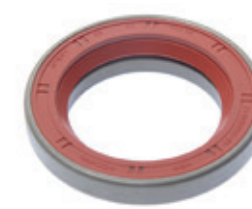
Артикул 21-1005032-01 Наименование Сальник коленвала ГАЗ-24, 53 в обойме 55x80x10
