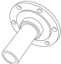
Артикул 230-12-007 Наименование Цапфа КАМАЗ кулака поворотного правая Cross № • 43114-2304078
