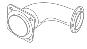
Артикул 120-14-051 Наименование Труба приемная глушителя КАМАЗ-6460 левая Cross № • 6460-1203014-40
