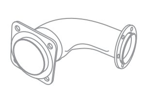
Артикул 120-14-054 Наименование Труба приемная глушителя КАМАЗ-65115 правая Cross № • 65115-1203013-12
