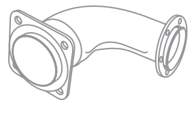
Артикул 120-14-063 Наименование Труба приемная глушителя КАМАЗ-6520 правая Cross № • 6522-1203013
