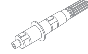
Артикул 170-16-069 Наименование Вал КПП ЗИЛ-130 первичный z=20
