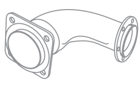
Артикул 120-14-059 Наименование Труба приемная глушителя КАМАЗ-6520 Cross № • 6520-1203011-04
