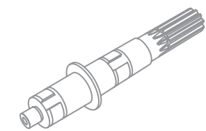
Артикул 170-16-009 Наименование Вал КПП УАЗ вторичный 4-х синхронной
