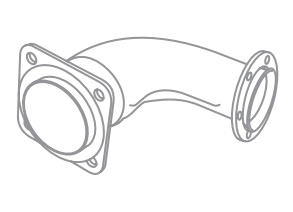
Артикул 120-14-068 Наименование Труба приемная глушителя КАМАЗ-65222 правая Cross № • 65222-1203013
